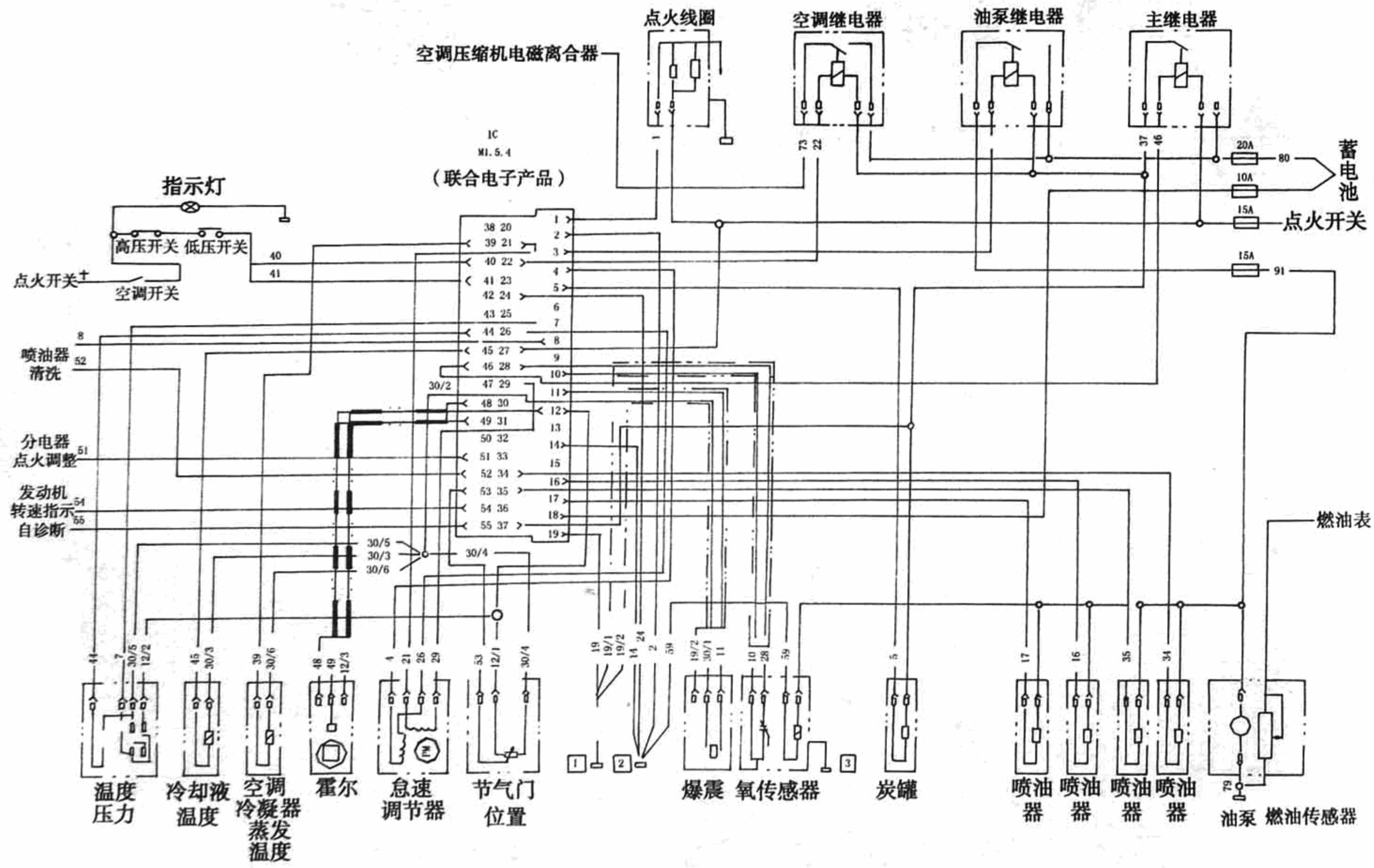
联合电子电控系统电路图
